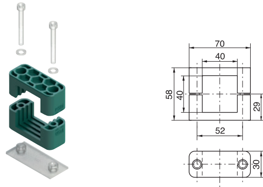
1 Stück = 2 Schellenhälften 1 piece = 2 clamp halves
